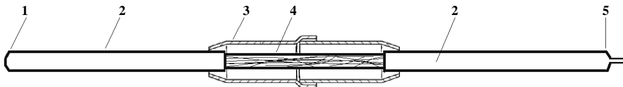
Рис. 1. Макет для пайки свинцовой муфты:
