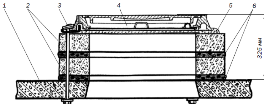
Рис. 15. Крепление опорных колец и люка с помощью «СНКЛ-3»:
