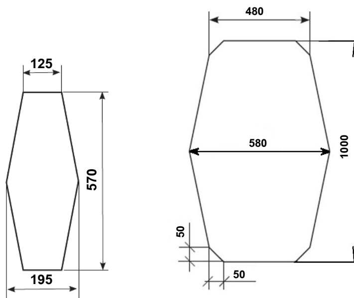
Рис. 2.2. Размеры технологического отверстия (слева) и участка с тонкой неармированной стенкой на торцевой стене колодца «ККСр-4-10».
