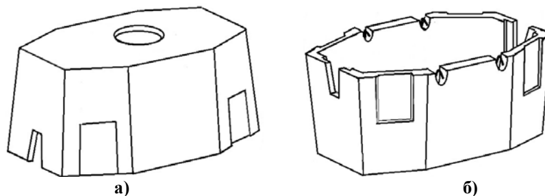
Рис. 1. Колодец «ККСр-4-10» как изделие по ТУ 45 1418-83: а – верхний элемент; б – нижний элемент.
