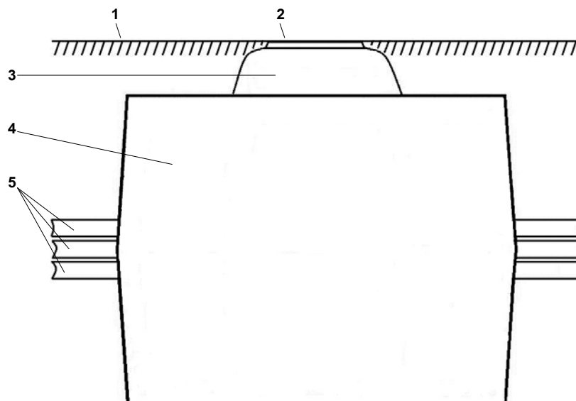
Рис. 2. Колодец «ККСр-4-10» как подземное сооружение: 1 – уровень земли или асфальта; 2 – чугунный люк; 3 – бетонная обмазка горловины; 4 – корпус колодца в сборе; 5 – вводимые каналы, 12 труб.
