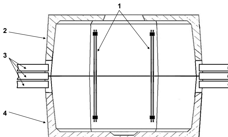
Рис. 10. Ввод труб в колодец «ККСр-4-10»:
