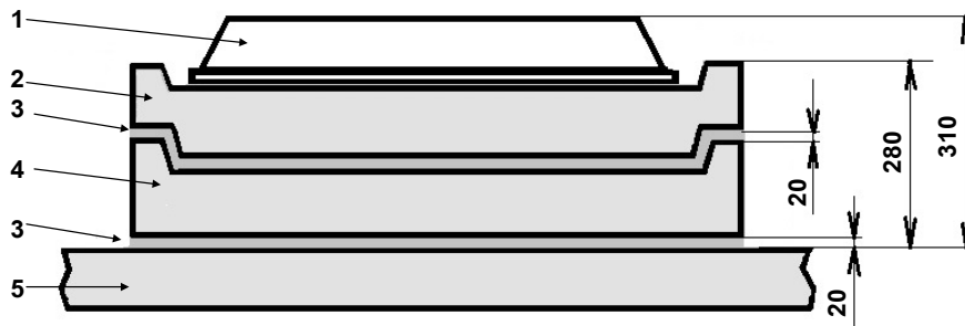
Рис. 13. Высота горловины с парой колец КО-ЧП и КО-Ч:
