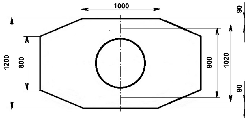
Рис. 6. Размеры перекрытия колодца «ККСр-4-10».
