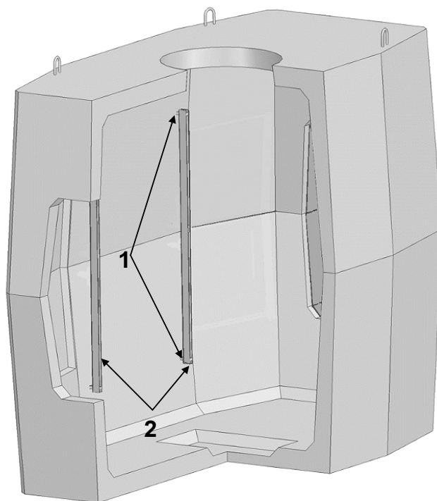
Рис. 3.1. Кронштейны «ККП-130» на боковой стене колодца «ККСр-4-10»: 1 – кронштейны; 2 – ерши с резьбой.
