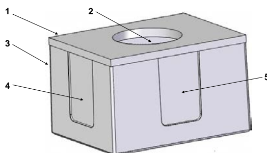
Рис. 3. Элементы на колодце «ККСр-1-10(80)» в сборе: 1 – плита перекрытия; 2 – круглое отверстие для люка; 3 – корпус; 4 – ниша на торцевой стене; 5 – ниша на боковой стене. Диаметр круглого отверстия для входного люка – 600 мм.
