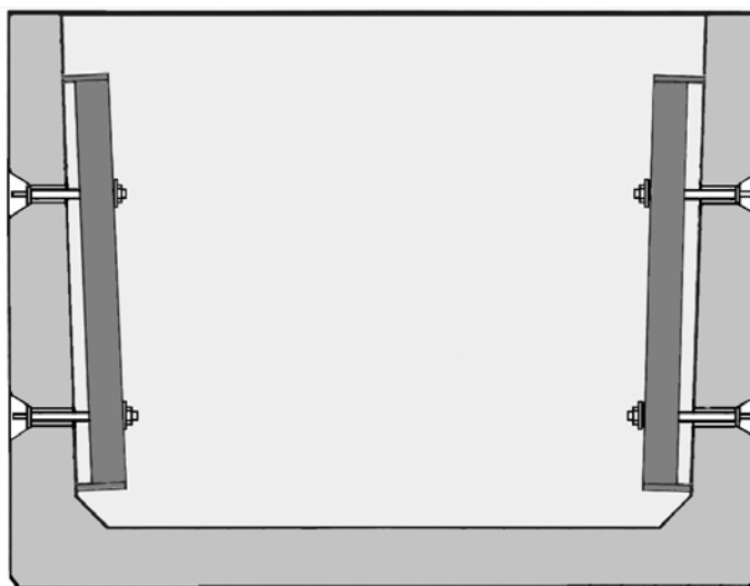
Рис. 2.2. Поперечный разрез колодца ККСр-1-10(80) с кронштейнами «ККП-60».
