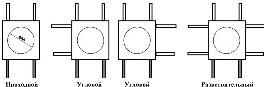
Рис. 7. Варианты использования колодца «ККСр-1-10(80)» в новых вариантах (для оптических кабелей).
