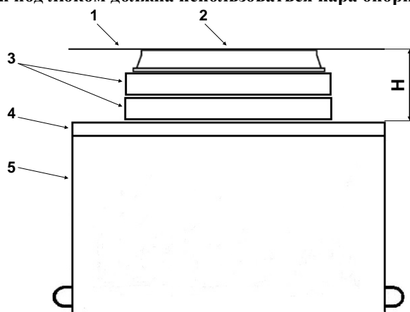
Рис. 7. Заглубление колодца «ККСр-1-10(80)» при установке на проезжей части:
