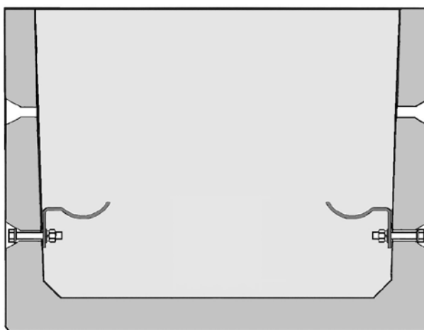
Рис. 2.1. Поперечный разрез колодца ККСр-1-10(80) с консолями «КСО-1».
