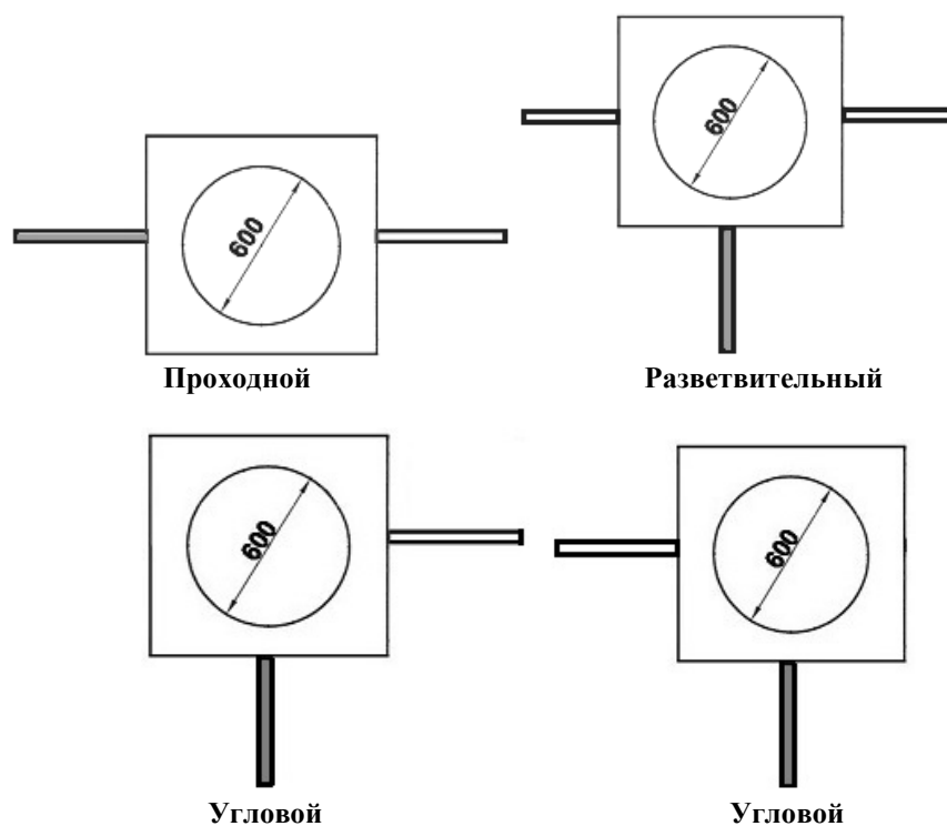
Рис. 6. Варианты использования колодца «ККСр-1-10(80)» в классических вариантах (для кабелей с медными жилами).
