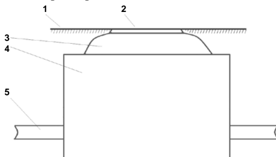
Рис. 5. Колодец «ККСр-1-10(80)» как подземное сооружение: 1 – уровень земли или дорожного покрытия; 2 – люк чугунный; 3 – горловина в бетонной обмазке; 4 – колодец в сборе (корпус + плита); 5 – вводимый канал.
