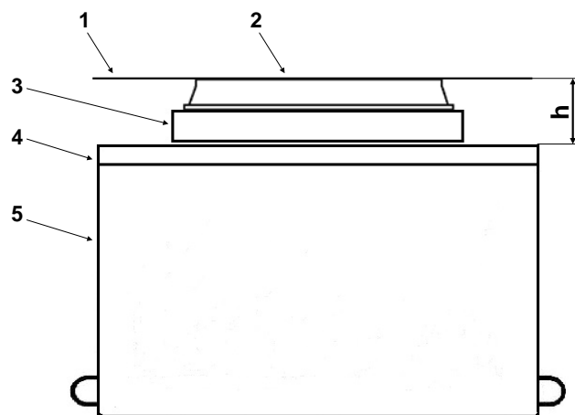
Рис. 6. Заглубление колодца «ККСр-1-10(80)» при установке на тротуаре или газоне:
