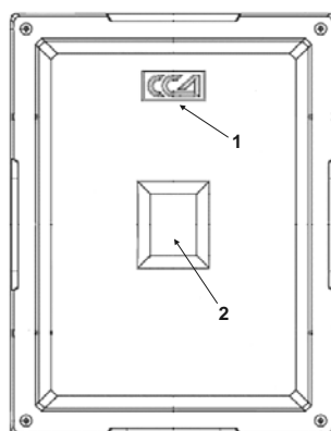
Рис. 2. Вид сверху на корпус колодца «ККСр-1-10(80)»: 1 – логотип компании ССД; 2 – приямок для стока воды.
