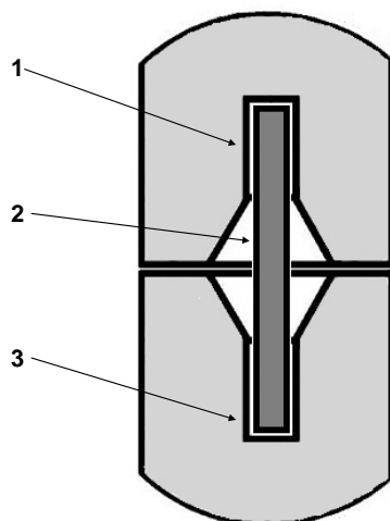
Рис. 11. Стержень в соединённых элементах колодца: 1 – углубление в верхнем элементе колодца; 2 – стальной стержень; 3 – углубление в нижнем элементе колодца.
