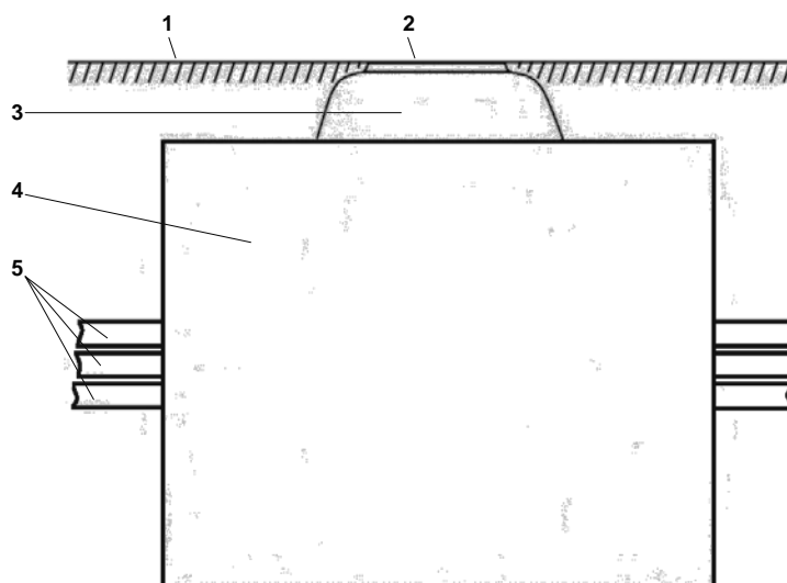
Рис. 6. Колодец «ККСр-3,5-10» как подземное сооружение: 1 – уровень земли или дорожного покрытия; 2 – люк чугунный; 3 – горловина в бетонной обмазке; 4 – колодец в сборе; 5 – вводимые каналы.
