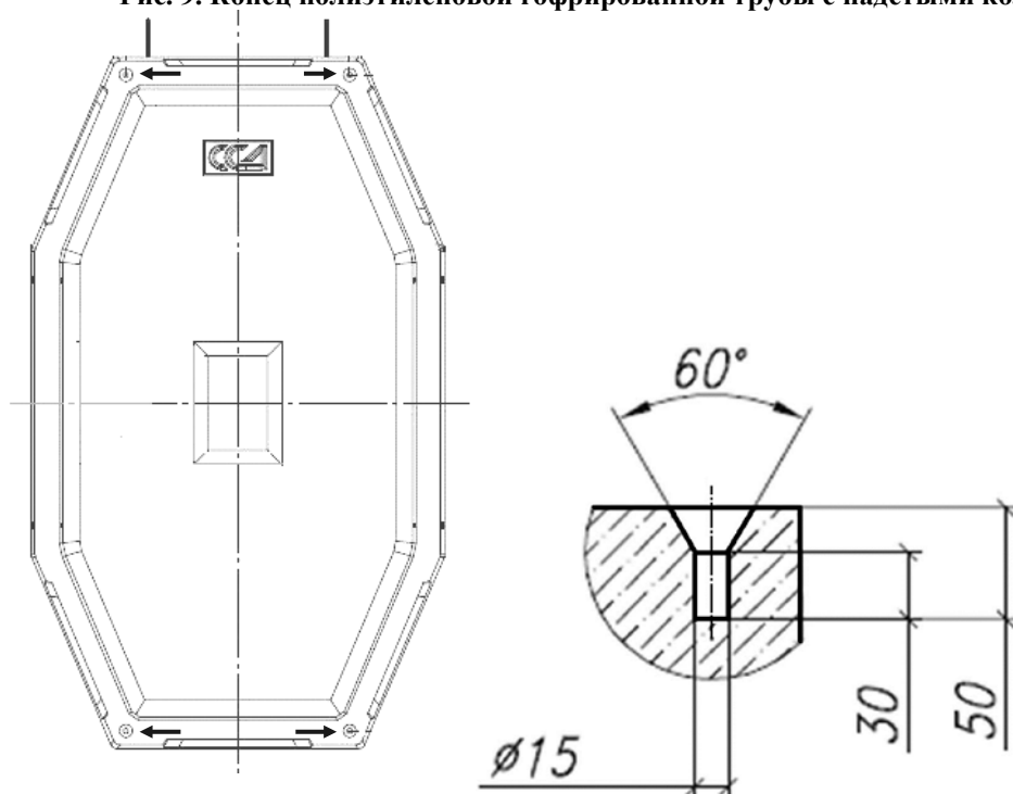
Рис. 10. Углубления для стержней на углах элемента колодца и форма углубления. Углубления показаны стрелками.
