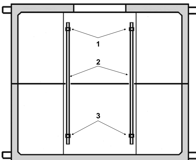
Рис. 3.4. Боковая стена колодца «ККСр-3,5-10» с установленными кронштейнами «ККП-130». 1 – ерши в верхних отверстиях верхнего элемента колодца; 2 – кронштейны «ККП-130»; 3 – ерши в нижних отверстиях нижнего элемента.
