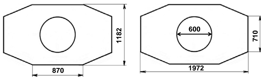
Рис. 4. Размеры перекрытия колодца «ККСр-3,5-10».
