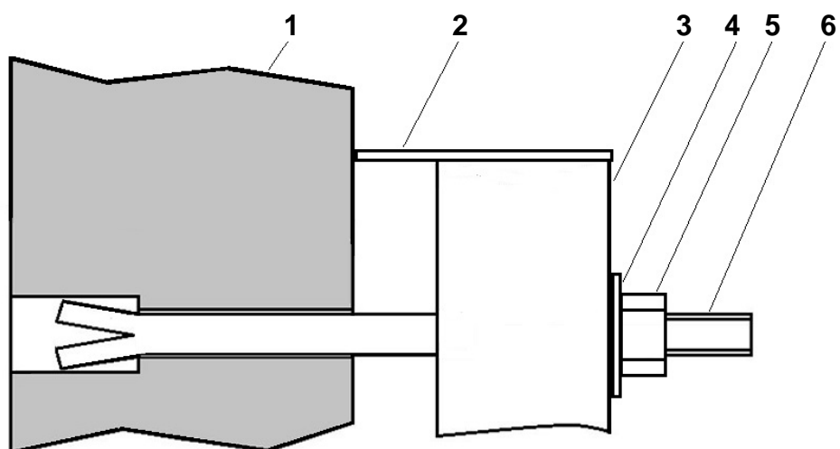
Рис. 3.3. Крепление кронштейна «ККП-130» на стене колодца «ККСр-3,5-10»: 1 – стена колодца; 2 – упор кронштейна; 3 – кронштейн ККП-130; 4 – квадратная шайба; 5 – гайка М12; 6 - резьбовая часть ерша, резьба М12.
