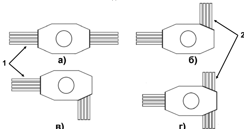
Рис. 7. Варианты использования колодца «ККСр-3,5-10»: а – проходной колодец; б и в – угловые колодцы; г – разветвительный колодец; 1 – вводимые каналы; 2 – ответвляющиеся каналы.
