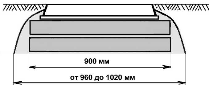
Рис. 13. Размеры (диаметры) опорных колец типа «КО» и бетонной обмазки.
