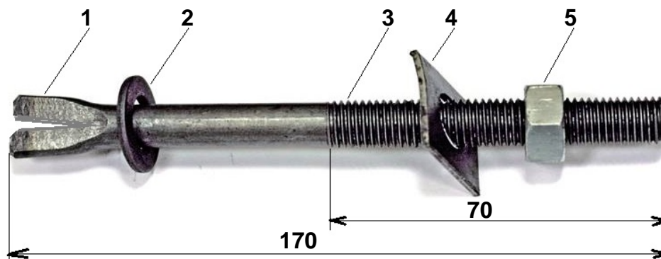
Рис. 3.2. Форма, размеры и дополнительные элементы ерша для крепления кронштейнов: 1 – расщепленный конец ерша (ласточкин хвост); 2 – круглая шайба; 3 – резьба М12; 4 – квадратная шайба; 5 – гайка М12.
