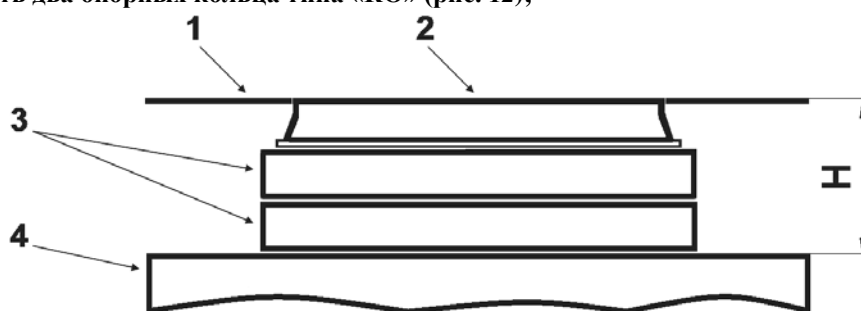
Рис. 12. Заглубление колодца «ККСр-3,5-10» при установке на тротуаре или газоне, вид на колодец сбоку: 1 – уровень тротуара или земли; 2 - люк чугунный лёгкого типа 3 – два опорных кольца; 4 – верхний элемент колодца; H – не менее 250 мм.
