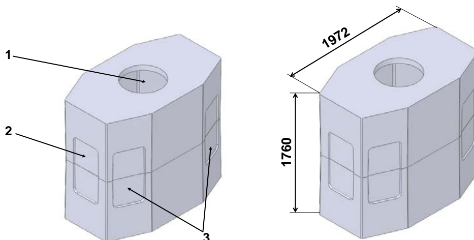
Рис. 3. Детали и габаритные размеры колодца «ККСр-3,5-10» в сборе: 1 – круглое отверстие для люка, диаметр 600 мм; 2 – ниша на торцевой стене верхнего элемента; 3 – ниши на боковых стенах элементов.
