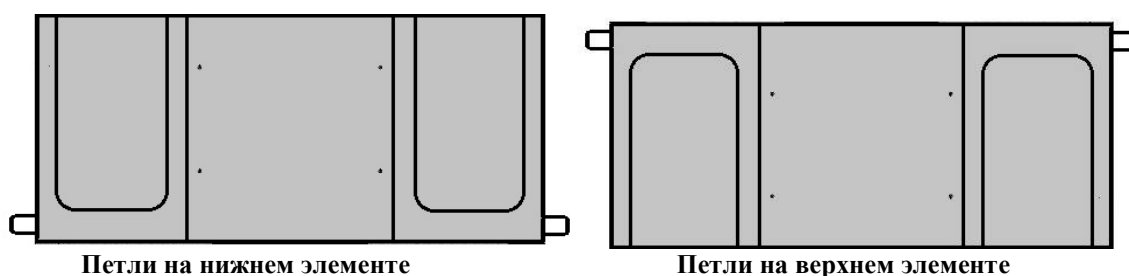
Рис. 8. Вид сбоку на элементы колодца «ККСр-3,5-10». Показаны места выхода подъёмных петель.
