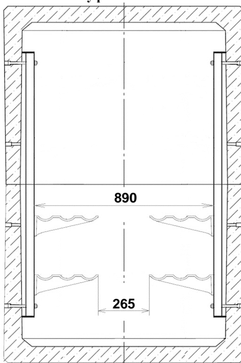
Рис. 4.1. Трёхместные консоли ККЧ-3 в колодце «ККСр-3,5-10».
