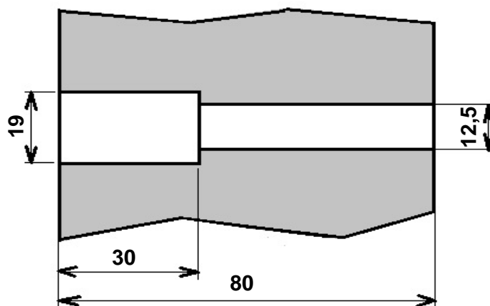
Рис. 3.1. Форма и размеры отверстий для ершей в стенах колодца «ККСр-3,5-10». Слева – наружная сторона стены, справа – внутренняя сторона стены.
