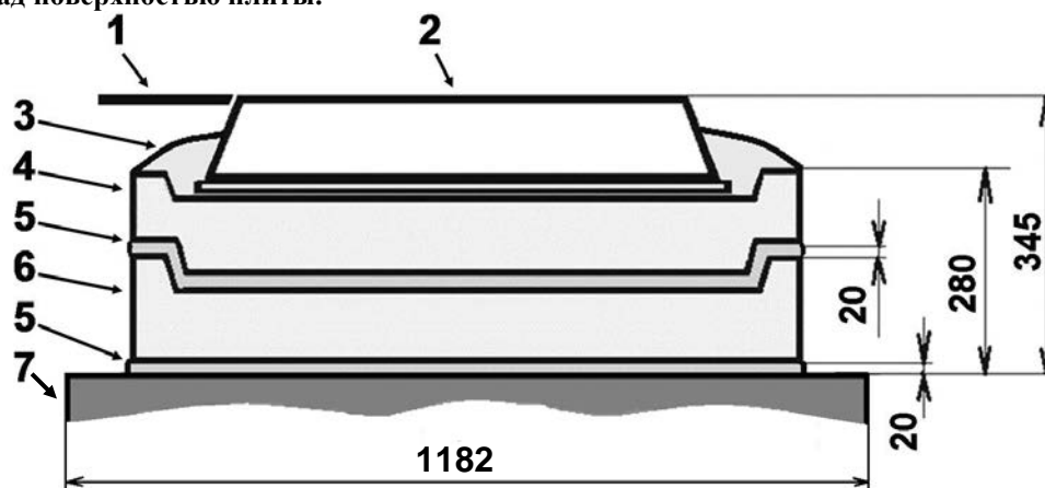
Рис. 14. Высота горловины с парой колец «КО-ЧП» и «КО-Ч», вид на колодец с торцевой стены:
