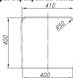
Рис. 5. Размеры ниш на верхнем элементе колодца «ККСр-3,5-10».
