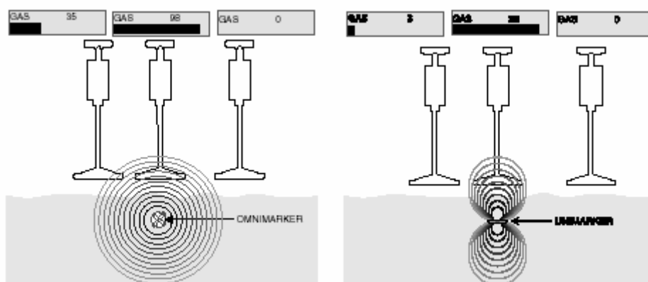
Рис. 32. Сигнал маркера Omni Marker Рис. 33. Сигнал маркера Uni Marker
