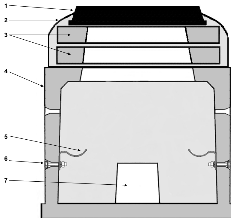
Рис. 1.1. Установка консолей типа КСО-1: 1 – чугунный люк для колодцев ГТС; 2 – бетонная обмазка; 3 – опорные кольца; 4 – боковая стена «ККСр-1М»; 5 – консоль типа КСО-1; 6 – болт с гайками и шайбами; 7 – отверстие для ввода трубы.
