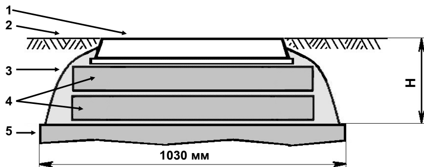
Рис. 8. Расстояние от перекрытия колодца до уровня асфальта на проезжей части: «H» – не менее 330 мм;
