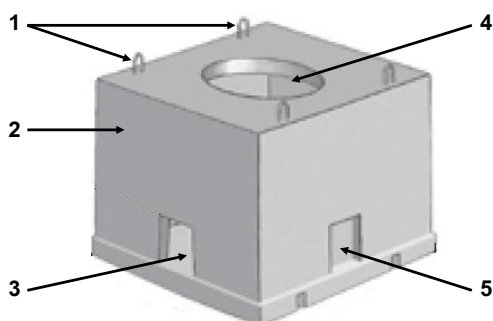
Рис. 1. Элементы колодца «ККСр-1М-10(80)» (монолитного): 1 – пегли; 2 – монолитный корпус; 3 - отверстие для ввода трубы; 4 – круглое отверстие для входного люка, диаметр 600 мм; 5 – ниша на боковой стене.
