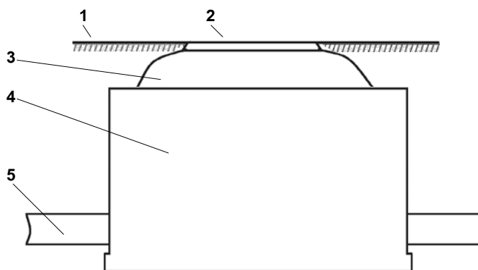
Рис. 2. Колодец «ККСр-1М-10(80)» как подземное сооружение: 1 – уровень земли или дорожного покрытия; 2 – люк чугунный; 3 – горловина в бетонной обмазке; 4 – колодец (монолитный корпус); 5 – вводимый канал.
