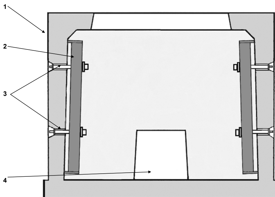
Рис. 1.2. Установка кронштейнов типа ККП-60: 1 – боковая стенка колодца «ККСр-1М»; 2 – кронштейн «ККП-60»; 3 – ерши с резьбой, с гайками и шайбами; 4 – отверстие для ввода трубы.
