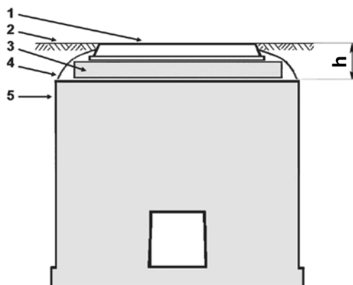
Рис. 7. Заглубление колодца «ККСр-1М» при установке на тротуаре или газоне: 1 – чугунная крышка люка; 2 – уровень тротуара или земли; 3 – одно опорное кольцо; 4 – бетонная обмазка; 5 – корпус колодца; h – не менее 100 мм.
