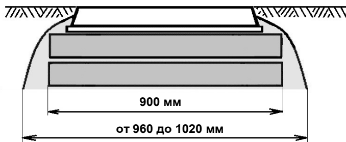
Рис. 9. Размеры (диаметры) опорных колец типа «КО» и бетонной обмазки.
