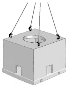
Рис. 5. Строповка колодца «ККСр-1М-10(80)».
