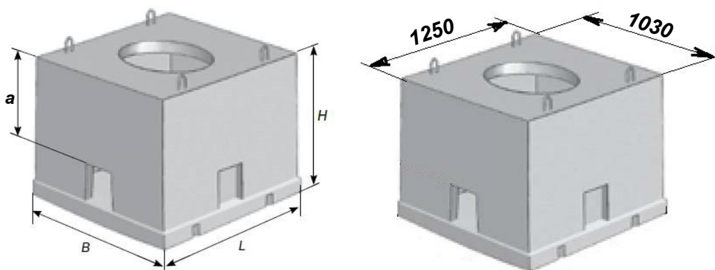
Рис. 3. Размеры колодца «ККСр-1М-10(80)» (монолитного).
