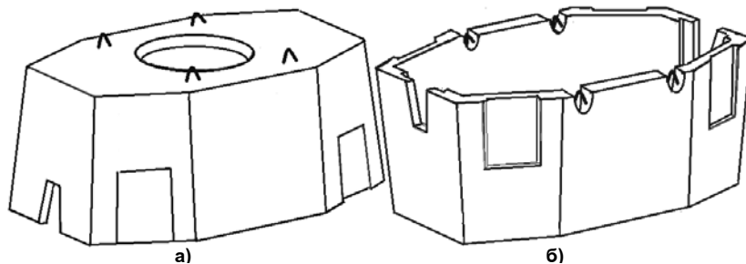
Рис. 1. Колодец «ККСр-3-10», как изделие по ТУ 45 1418-83: а – верхний элемент колодца; б - нижний элемент.
