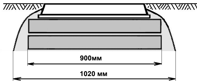
Рис. 13. Размеры (диаметры) опорных колец типа КО и бетонной обмазки. Вид на колодец «ККСр-3-10» сбоку.
