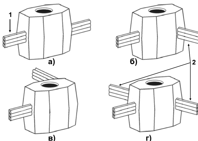
Рис. 3. Варианты использования колодца «ККСр-3-10»: 1 – вводимые каналы; 2 – ответвляющиеся каналы; а - проходной колодец; б, в – угловые колодцы; г - разветвительный колодец.
