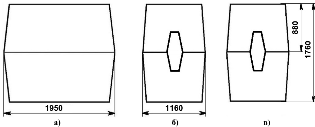
Рис. 5. Габаритные размеры колодца «ККСр-3-10»:
