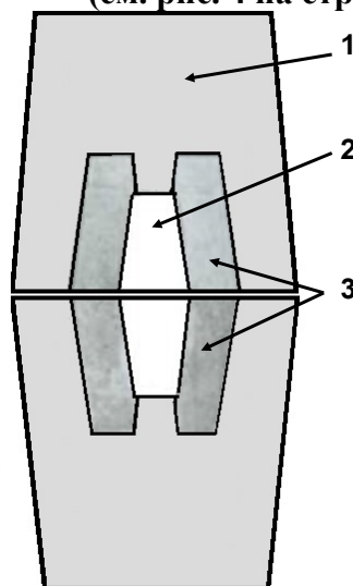
Рис. 2.1. Форма участка с тонкой неармированной стенкой на внутренней поверхности торцевой стены колодца «ККСр-3-10»:
