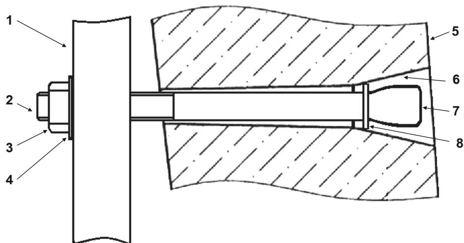
Рис. 3.3. Крепление кронштейна типа ККП с помощью ершей с резьбой: 1 – кронштейн ККП; 2 – ёрш, конец с резьбой М12; 3 – гайка М12; 4 – шайба; 5 – боковая стена колодца; 6 – отверстие для ерша; 7 – ёрш, расплющенный конец; 8 – шайба.
