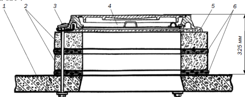
Рис. 14. Крепление опорных колец и люка с помощью «СНКЛ-3»: 1 – перекрытие колодца; 2 – кольца КО-1; 3 – набор «СНКЛ-3»; 4 – люк чугунный лёгкого типа; 5 – слой строительного раствора; 6 – слой бетона.
