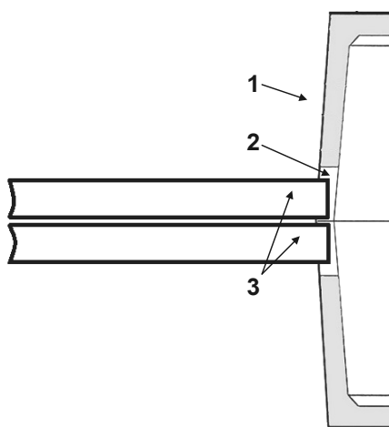
Рис. 10. Ввод труб в колодец «ККСр-3-10»:
