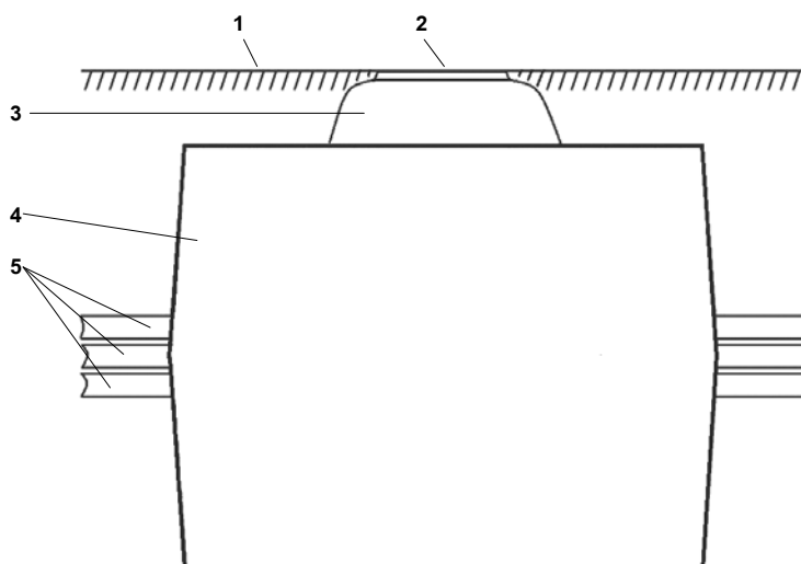
Рис. 2. Колодец «ККСр-3-10», как подземное сооружение: 1 – уровень земли или асфальта на тротуаре; 2– чугунный люк лёгкого типа; 3 – горловина в бетонной обмазке; 4 – корпус (верхний и нижний элементы); 5 – блок вводимых каналов.
