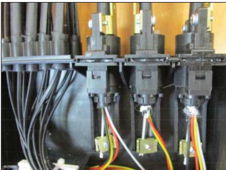
Рисунок А2 – Введенные ОК в муфту-красса
