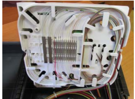
Рисунок А4 – Общий вид внутренней части кассеты
