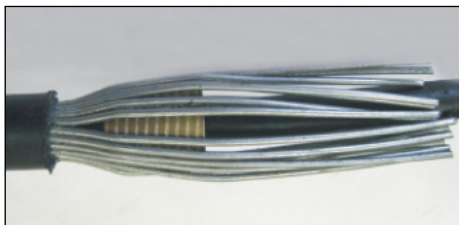
5.2 Обжать стальные проволоки брони вокруг внутреннего конуса.
