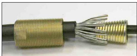
5.4 Продвинуть конус обратно на внутреннюю оболочку и отогнуть стальные проволоки на 10-12°. Вдавить обратно конус до упора и снова обжать его проволоками брони.
