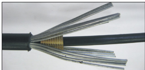
5.1 Надвинуть внутренний конус на внутреннюю оболочку кабеля до упора.
