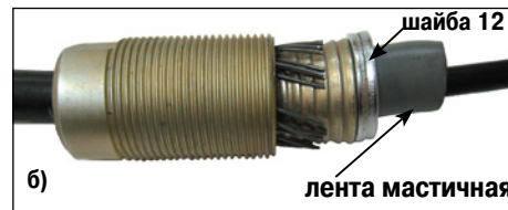
5.3 Обрезать проволоки по окружности на расстоянии 2/3 длины конуса.
