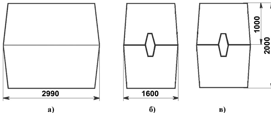
Рис. 5. Габаритные размеры колодца «ККСр-5-10»: а - вид сбоку; б и в – виды с торца.
