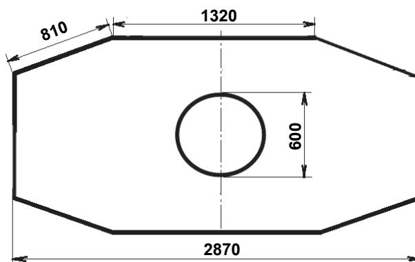
Рис. 6. Размеры перекрытия колодца «ККСр-5-10».
