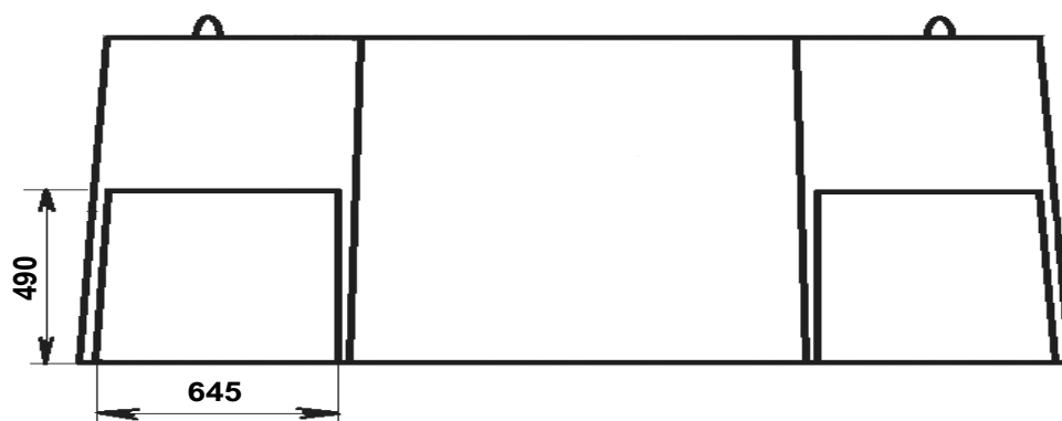
Рис. 8. Размеры ниш на примере верхнего элемента колодца «ККСр-5-10». На нижнем элементе ниши такого же размера.
