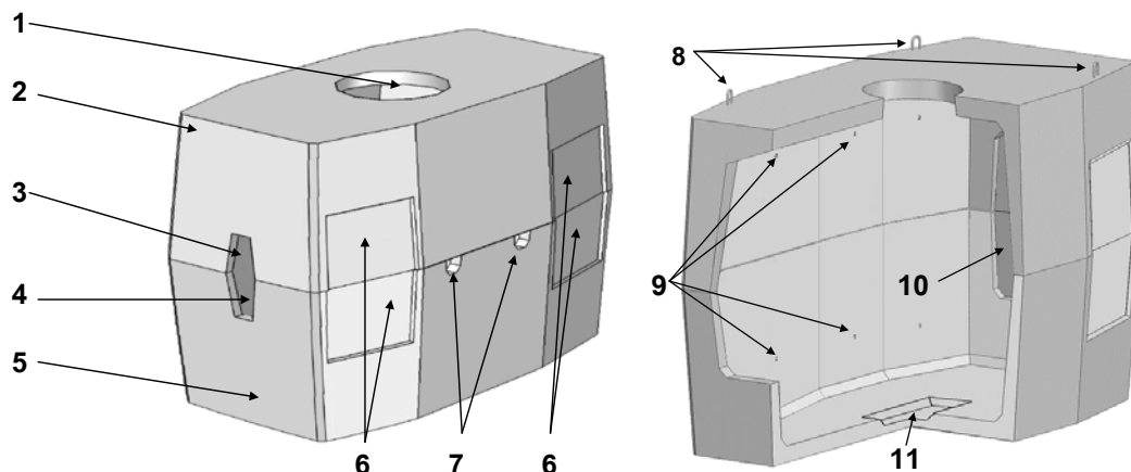
Рис. 4. Колодец «ККСр-5-10», внешний вид и детали элементов колодца: 1 – круглое отверстие для люка; 2 – верхний элемент; 3 – технологическое отверстие верхнего элемента; 4 – технологическое отверстие нижнего элемента; 5 – нижний элемент; 6 – ниши на наружных поверхностях боковых стен; 7 – гнезда с подъёмными петлями на нижнем элементе; 8 – подъёмные петли на перекрытии; 9 – отверстия для ершей; 10 – участки с тонкой неармированной стенкой вокруг технологических отверстий в элементах; 11 – приямок для стока воды.
