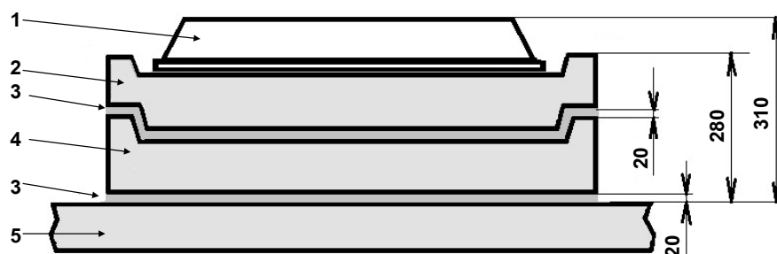
Рис. 13. Высота горловины с парой колец КО-ЧП и КО-Ч: 1 – люк чугунный лёгкого типа; 2 – кольцо «КО-Ч»; 3 – слой бетона; 4 – опорное кольцо «КО-ЧП»; 5 – перекрытие колодца «ККСр-5-10».
