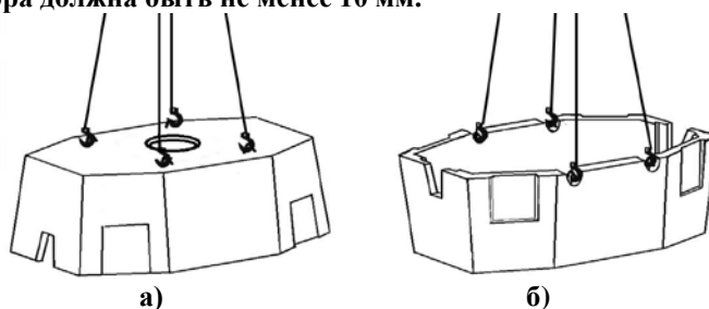
Рис. 9. Строповка элементов «ККСр-5-10»: а – верхнего элемента; б – нижнего элемента.
