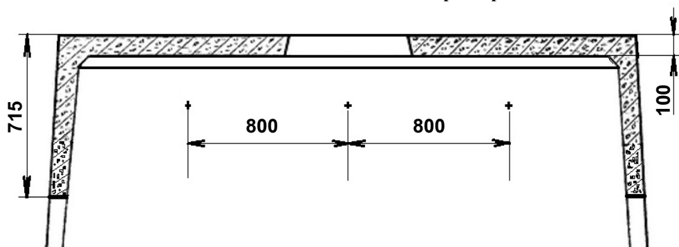
Рис. 9. Размеры колодца «ККСр-5-10» на продольном разрезе верхнего элемента: толщина перекрытия; расстояние от перекрытия до технологического отверстия; расстояние между отверстиями для ершей.
