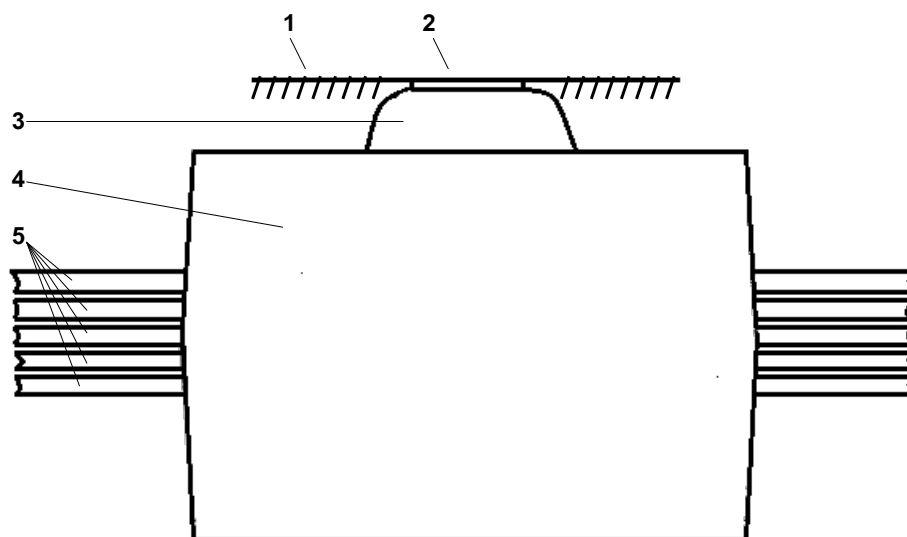
Рис. 2. Колодец «ККСр-5-10» как подземное сооружение: 1 – уровень земли или асфальта; 2 – чугунный люк; 3 – бетонная обмазка горловины; 4 – корпус колодца в сборе; 5 – вводимые каналы, 24 трубы.
