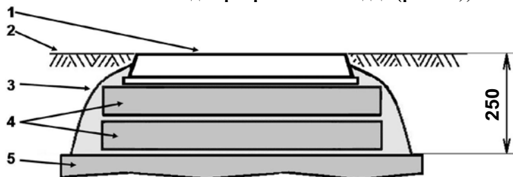
Рис. 12. Расстояние от перекрытия колодца до уровня земли (асфальта) на тротуаре и газоне должно быть – не менее 250 мм:
