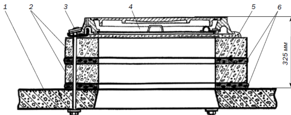
Рис. 15. Крепление опорных колец и люка с помощью «СНКЛ-3»: 1 – перекрытие колодца; 2 – кольца КО-1; 3 – набор «СНКЛ-3»; 4 – люк чугунный лёгкого типа; 5 – слой строительного раствора; 6 – слой бетона.
