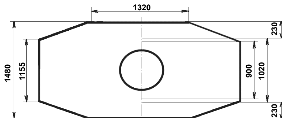
Рис. 7. Размеры перекрытия колодца «ККСр-5-10» с указанием диаметров опорных колец: 900 мм – кольца типа КО; 1020 мм – колец КО-ЧП и КО-Ч.
