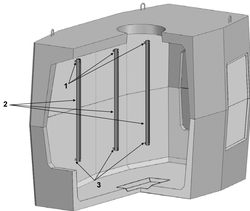
Рис. 3.1. Кронштейны «ККП-130» на боковой стене колодца «ККСр-5-10»: 1 – ерши в верхнем элементе; 2 - кронштейны; 3 – ерши в нижнем элементе.
