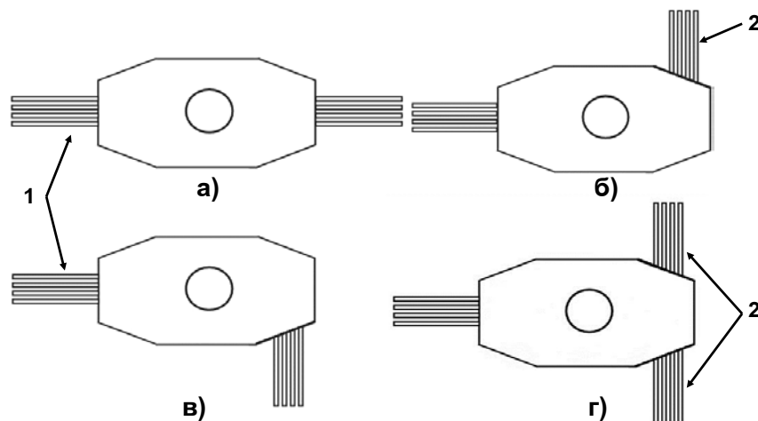
Рис. 3. Варианты использования колодца «ККСр-5-10»: 1 – вводимые каналы; 2 – ответвляющиеся каналы; а - проходной колодец; б, в – угловые колодцы; г - разветвительный колодец.
