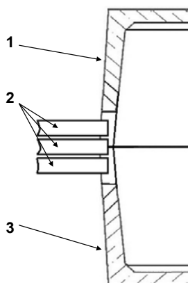
Рис. 10. Ввод труб в колодец «ККСр-5-10»:
