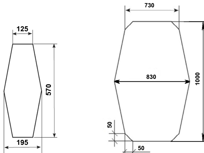
Рис. 2.2. Размеры технологического отверстия и участка с тонкой неармированной стенкой на торцевой стене колодца «ККСр-5-10».
