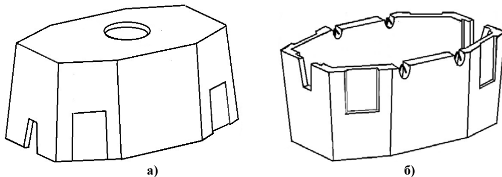
Рис. 1. Колодец «ККСр-5-10» как изделие по ТУ 45 1418-83: а – верхний элемент; б – нижний элемент.
