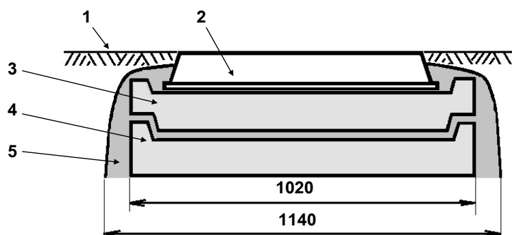
Рис. 14 Диаметры колец и обмазанной бетоном горловины при использовании пары «КО-ЧП» и «КО-Ч»: 1 – уровень земли на газоне, асфальта на тротуаре; 2 – люк лёгкого типа; 3 – кольцо «КО-Ч»; 4 – кольцо «КО-ЧП»; 5 - обмазка горловины бетоном со щебнем.
