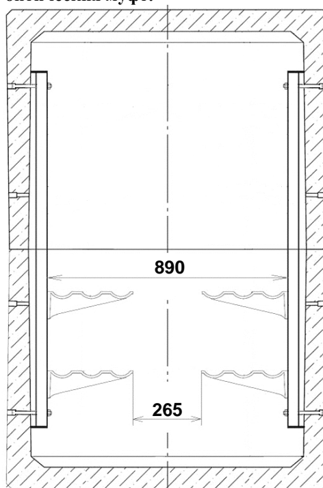
Рис. 4.1. Трёхместные консоли ККЧ-3 в колодце «ККСр-3,5-80».
