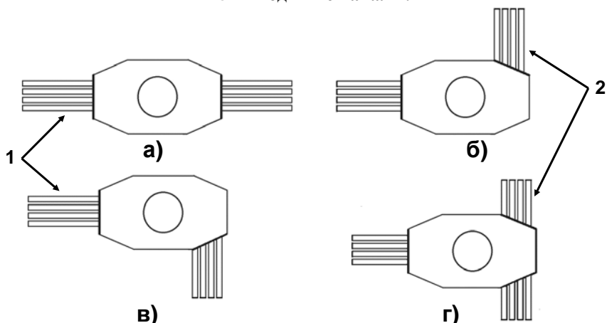
Рис. 7. Варианты использования колодца «ККСр-3,5-10(80)»: а – проходной колодец; б и в – угловые колодцы; г – разветвительный колодец; 1 – вводимые каналы; 2 – ответвляющиеся каналы.
