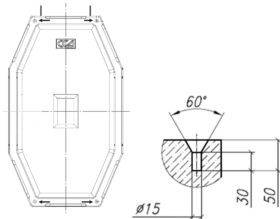
Рис. 10. Углубления для фиксаторов смещения на углах элемента колодца и форма углубления. Углубления показаны стрелками.
