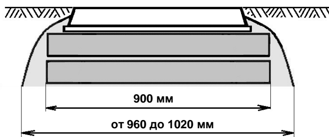
Рис. 13. Размеры (диаметры) опорных колец типа «КО» и бетонной обмазки.
