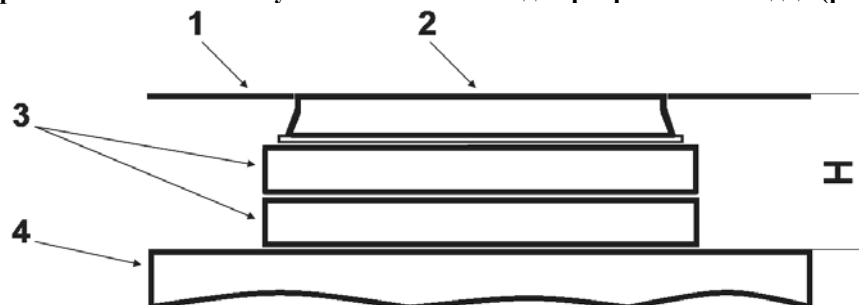
Рис. 12. Заглубление колодца «ККСр-3,5-10(80)» при установке на тротуаре или газоне, вид на колодец сбоку:
