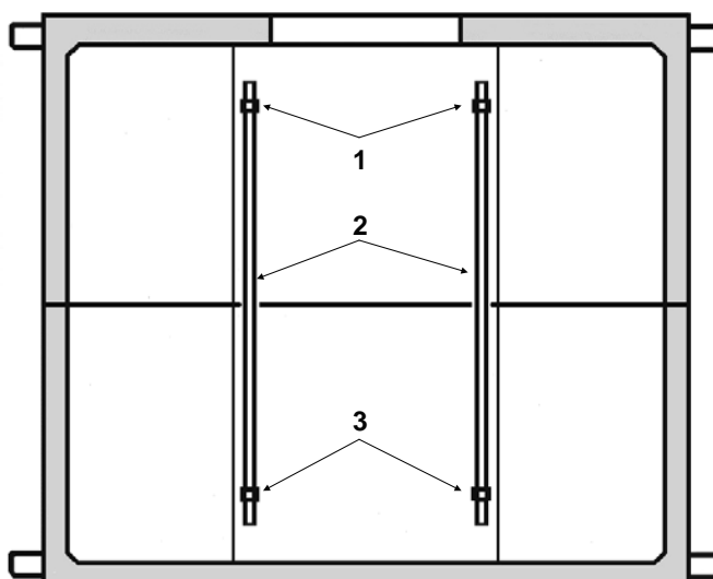
Рис. 3.4. Боковая стена колодца «ККСр-3,5-10(80)» с установленными кронштейнами «ККП-130». 1 – ерши в верхних отверстиях верхнего элемента колодца; 2 – кронштейны «ККП-130»; 3 – ерши в нижних отверстиях нижнего элемента.
