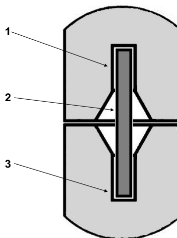
Рис. 11. Фиксатор смещения в соединённых элементах колодца: 1 – углубление в верхнем элементе колодца; 2 – фиксатор смещения; 3 – углубление в нижнем элементе колодца.
