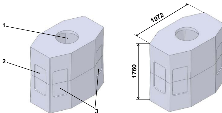
Рис. 3. Детали и габаритные размеры колодца «ККСр-3,5-10(80)» в сборе: 1 – круглое отверстие для люка, диаметр 600 мм; 2 – ниша на торцевой стене верхнего элемента; 3 – ниши на боковых стенах элементов.
