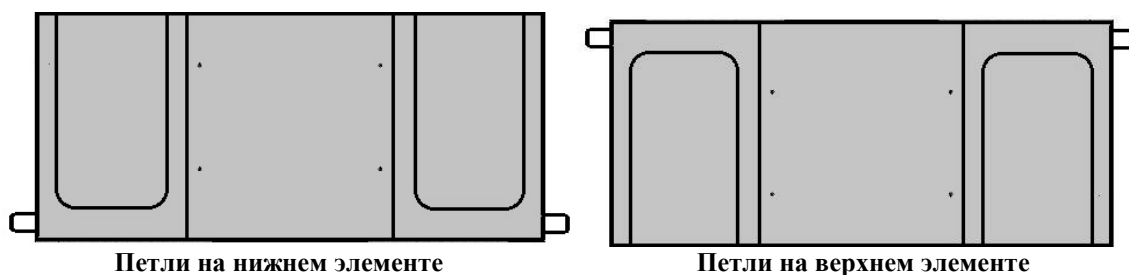
Рис. 8. Вид сбоку на элементы колодца «ККСр-3,5-10(80)». Показаны места выхода подъёмных петель.
