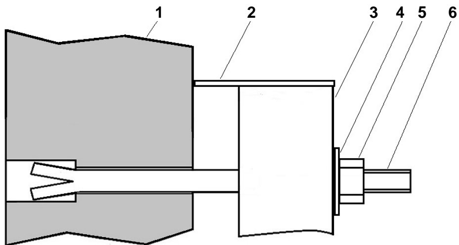
Рис. 3.3. Крепление кронштейна «ККП-130» на стене колодца «ККСр-3,5-10(80)»: 1 – стена колодца; 2 – упор кронштейна; 3 – кронштейн ККП-130; 4 – квадратная шайба; 5 – гайка М12; 6 – резьбовая часть ерша, резьба М12.
