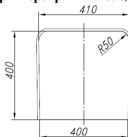
Рис. 5. Размеры ниш на верхнем элементе колодца «ККСр-3,5-10(80)». Ниши на нижнем элементе имеют те же размеры.
