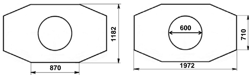
Рис. 4. Размеры перекрытия колодца «ККСр-3,5-10(80)».
