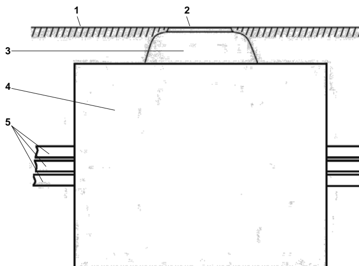
Рис. 6. Колодец «ККСр-3,5-10(80)» как подземное сооружение: 1 – уровень земли или дорожного покрытия; 2 – люк чугунный; 3 – горловина в бетонной обмазке; 4 – колодец в сборе; 5 – вводимые каналы.
