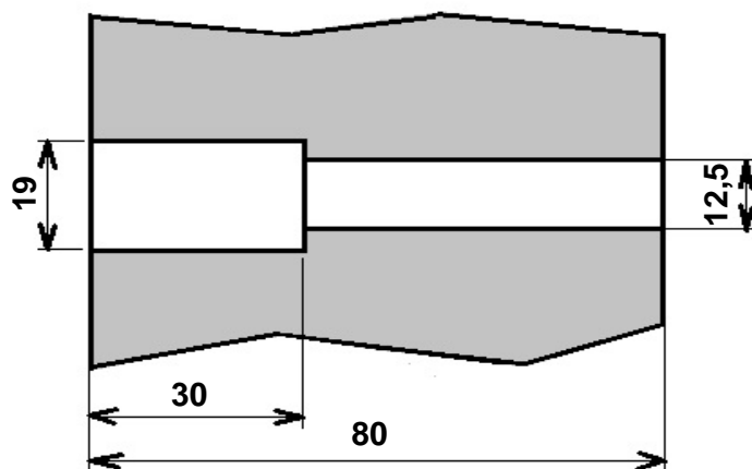
Рис. 3.1. Форма и размеры отверстий для ершей в стенах колодца «ККСр-3,5-80». Слева – наружная сторона стены, справа – внутренняя сторона стены.
