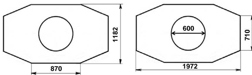
Рис. 4. Размеры перекрытия колодца «ККСр-3,5-80».
