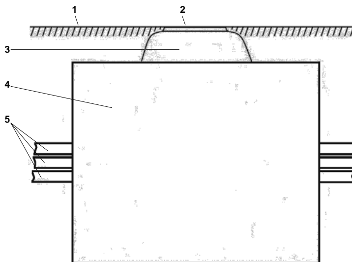
Рис. 6. Колодец «ККСр-3,5-80» как подземное сооружение: 1 – уровень земли или дорожного покрытия; 2 – люк чугунный; 3 – горловина в бетонной обмазке; 4 – колодец в сборе; 5 – вводимые каналы.
