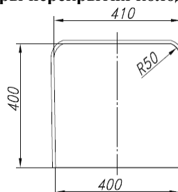
Рис. 5. Размеры ниш на верхнем элементе колодца «ККСр-3,5-80».
