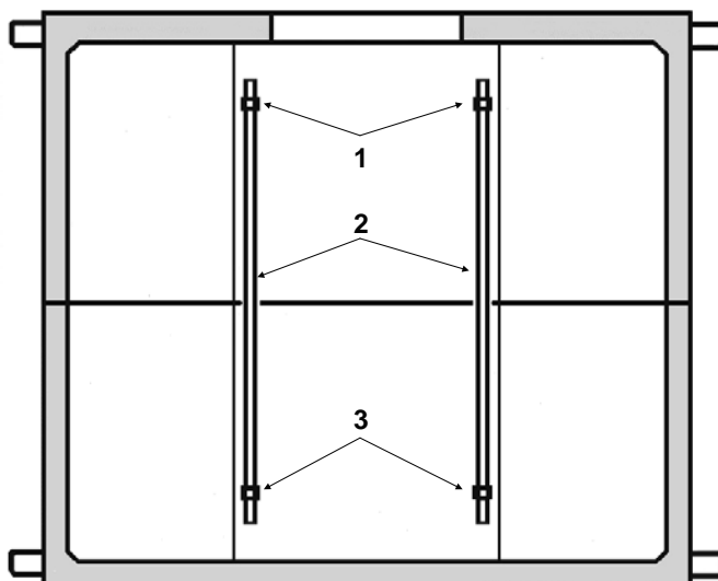
Рис. 3.4. Боковая стена колодца «ККСр-3,5-80» с установленными кронштейнами «ККП-130». 1 – ерши в верхних отверстиях верхнего элемента колодца; 2 – кронштейны «ККП-130»; 3 – ерши в нижних отверстиях нижнего элемента.
