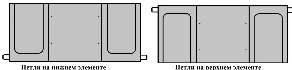
Рис. 8. Вид сбоку на элементы колодца «ККСр-3,5-80». Показаны места выхода подъёмных петель.
