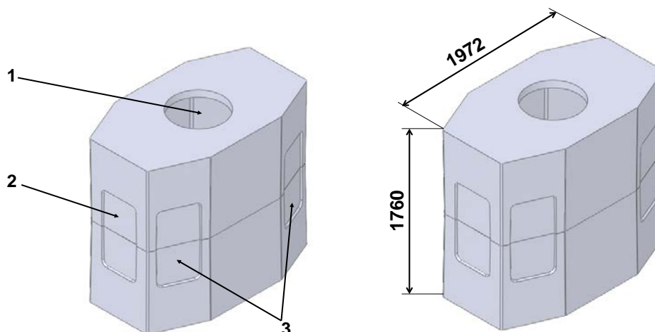
Рис. 3. Детали и габаритные размеры колодца «ККСр-3,5-80» в сборе: 1 – круглое отверстие для люка, диаметр 600 мм; 2 – ниша на торцевой стене верхнего элемента; 3 – ниши на боковых стенах элементов.
