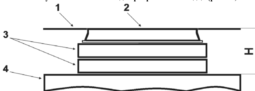
Рис. 12. Заглубление колодца «ККСр-3,5-80» при установке на тротуаре или газоне, вид на колодец сбоку:
