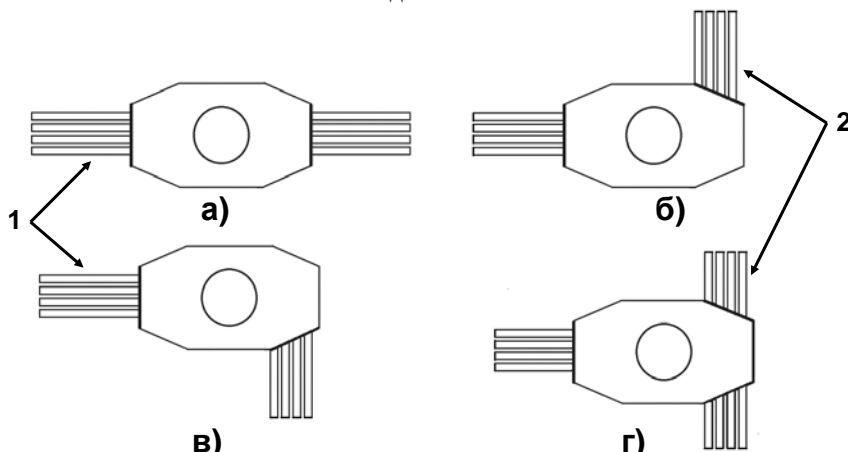
Рис. 7. Варианты использования колодца «ККСр-3,5-80»: а – проходной колодец; б и в – угловые колодцы; г – разветвительный колодец; 1 – вводимые каналы; 2 – ответвляющиеся каналы.
