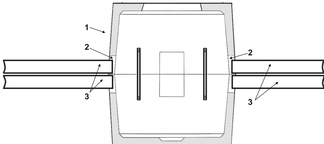
Рис. 9. Ввод труб в колодец «ККСр-2-10(80)»: 1 – торцевая стена колодца; 2 – проёмы в торцевых стенках; 3 – хризотилцементные (асбестоцементные) трубы.
