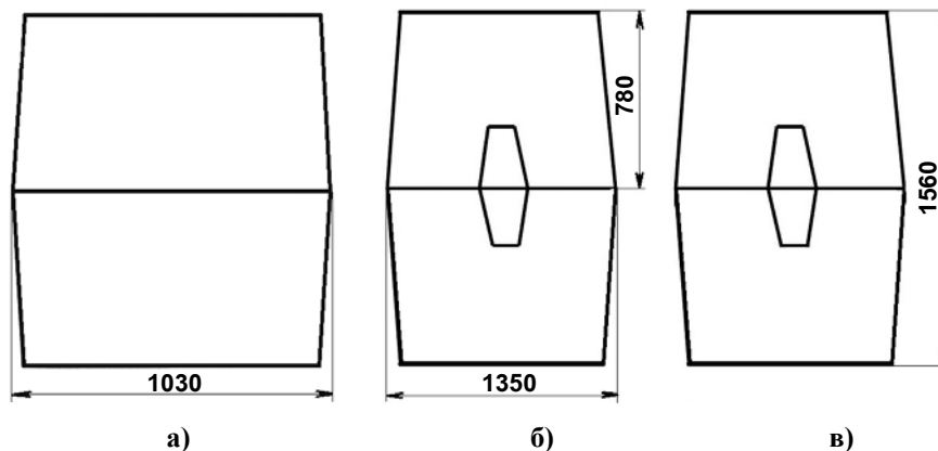
Рис. 6. Габаритные размеры колодца «ККСр-2-10(80)»: а - вид сбоку; б и в – вид с торца.
