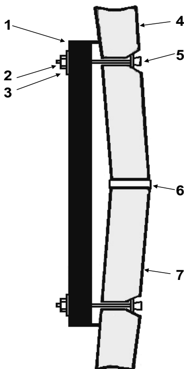
Рис. 3.2. Крепление кронштейна «ККП-60»: 1 – кронштейн «ККП-60»; 2 – гайка на ёрше; 3 – шайба; 4 – боковая стена верхнего элемента колодца; 5 – ёрш; 6 – слой строительного раствора между элементами колодца; 7 – боковая стена нижнего элемента колодца.
