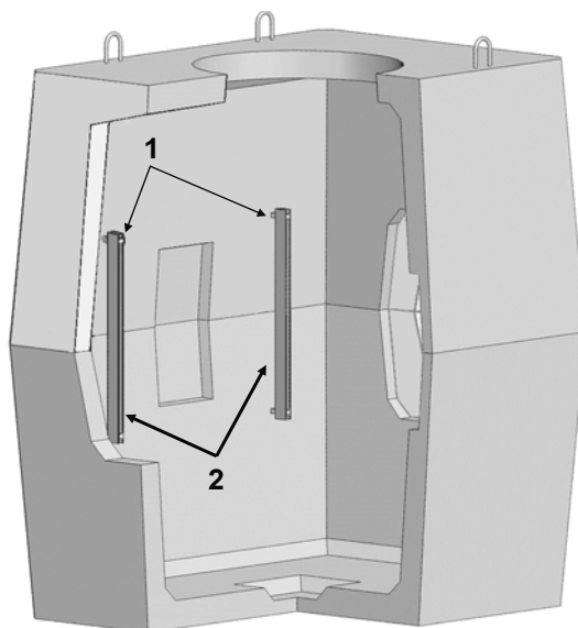
Рис. 3.1. Установка кронштейнов «ККП-60» в колодце «ККСр-2-10(80)»: 1 – ёрши с резьбой, гайками и шайбами; 2 – кронштейны «ККП-60».
