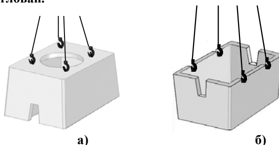
Рис. 8. Строповка элементов «ККСр-2-10(80)»: а – верхнего элемента; б – нижнего элемента.
