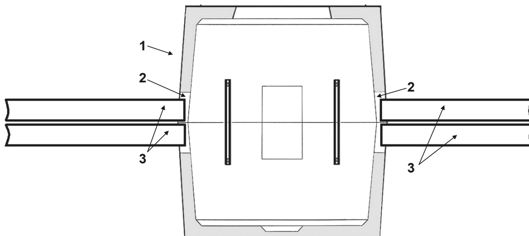
Рис. 9. Ввод труб в колодец «ККСр-2-10(80)»:
