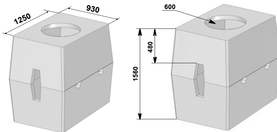
Рис. 5. Внешний вид колодца «ККСр-2-10(80)» с размерами. Диаметр круглого отверстия для люка - 600 мм.
