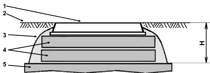
Рис. 11. Расстояние от перекрытия колодца до уровня земли (асфальта) – Н: на тротуаре и газоне – не менее 250 мм; на проезжей части – не менее 330 мм: 1 – люк чугунный; 2 – уровень земли на газоне, асфальта на тротуаре или дорожного покрытия на проезжей части улиц; 3 – обмазка бетоном со щебнем; 4 – опорные кольца типа КО; 5 – перекрытие колодца «ККСр-2-10(80)».
