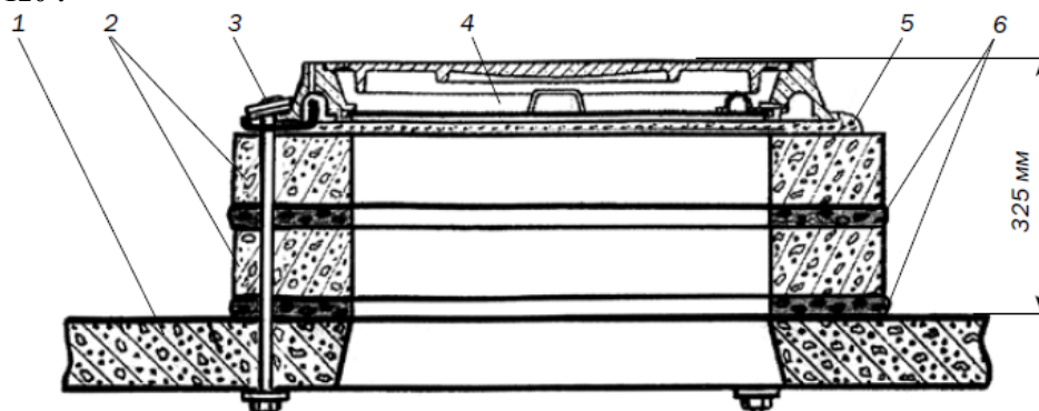
Рис. 13. Крепление опорных колец и люка с помощью «СНКЛ-3»: 1 – перекрытие колодца; 2 – кольца КО-1; 3 – набор «СНКЛ-3»; 4 – люк чугунный лёгкого типа; 5 – слой строительного раствора; 6 – слой бетона.
