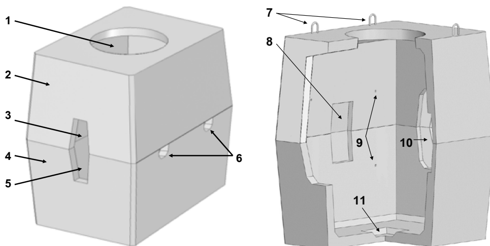
Рис. 4. Детали колодца «ККСр-2-10(80)»:
