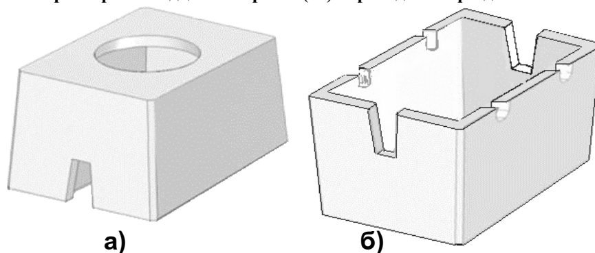
Рис. 1. Колодец «ККСр-2-10(80)» как изделие по ТУ 45 1418-83: а – верхний элемент; б – нижний элемент.
