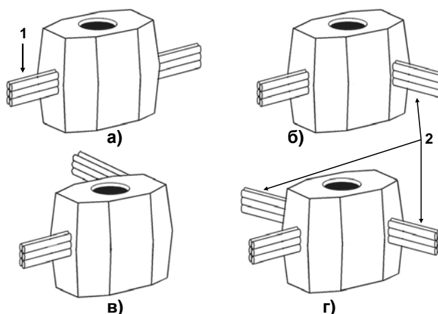
Рис. 3. Варианты использования колодца «ККСр-3М-10(80)»: 1 – вводимые каналы; 2 – ответвляющиеся каналы; а - проходной колодец; б, в – угловые колодцы; г - разветвительный колодец.
