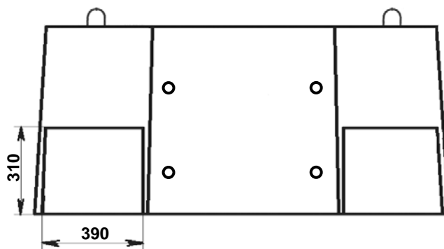
Рис. 8. Размеры ниш на примере верхнего элемента колодца «ККСр-3М-10(80)». На нижнем элементе ниши такого же размера.
