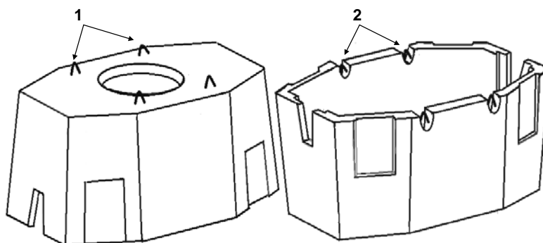
Рис. 5. Подъёмные петли на элементах колодца «ККСр-3М-10(80)»: 1 – петли на перекрытии верхнего элемента; 2 – петли в гнёздах на нижнем элементе.
