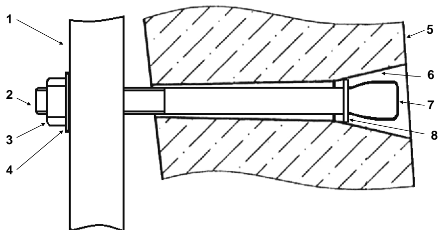
Рис. 3.2. Крепление кронштейна типа УККП с помощью ершей с резьбой: 1 – кронштейн УККП; 2 – ёрш, конец с резьбой М12; 3 – гайка М12; 4 – шайба; 5 – боковая стена колодца; 6 – отверстие для ерша; 7 – ёрш, расплющенный конец; 8 – шайба.
