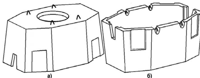
Рис. 1. Колодец «ККСр-3М-10(80)», как изделие по ТУ 45 1418-83: а – верхний элемент колодца; б - нижний элемент.
