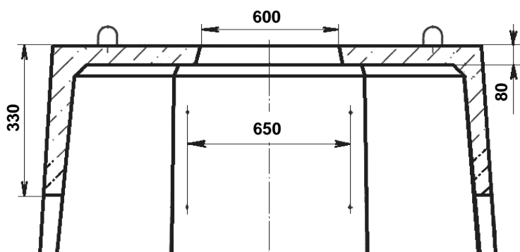
Рис. 9. Размеры колодца «ККСр-3М-10(80)» на продольном разрезе верхнего элемента: толщина перекрытия; расстояние от перекрытия до технологического отверстия; диаметр горловины; расстояние между отверстиями для ершей.
