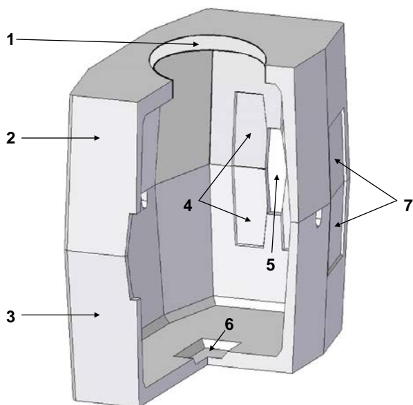
Рис. 4. Колодец «ККСр-3М-10(80)» в сборе, внешний вид и детали элементов колодца: 1 – круглое отверстие для люка; 2 – верхний элемент; 3 – нижний элемент; 4 – участки с тонкой неармированной стенкой вокруг технологических отверстий; 5 – технологические отверстия в элементах; 6 – приямок для стока воды; 7 – ниши на элементах.
