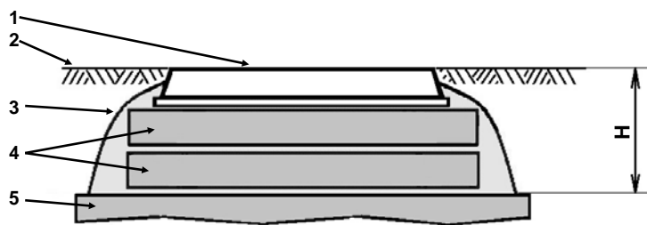
Рис. 13. Расстояние от перекрытия колодца до уровня земли (асфальта) – Н: на тротуаре и газоне – не менее 250 мм; на проезжей части – не менее 330 мм: 1 – люк чугунный; 2 – уровень земли на газоне, асфальта на тротуаре или дорожного покрытия на проезжей части улиц; 3 – обмазка бетоном со щебнем; 4 – опорные кольца типа КО; 5 – перекрытие колодца «ККСр-3М-10(80)».
