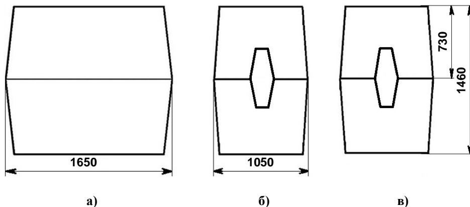
Рис. 6. Габаритные размеры колодца «ККСр-3М-10(80)»: а - вид сбоку; б и в – виды с торца.
