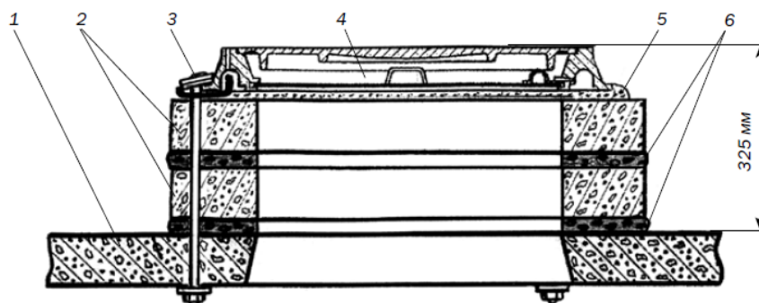
Рис. 15. Крепление опорных колец и люка с помощью «СНКЛ-3»: 1 – перекрытие колодца; 2 – кольца КО-1; 3 – набор «СНКЛ-3»; 4 – люк чугунного лёгкого типа; 5 – слой строительного раствора; 6 – слой бетона.
