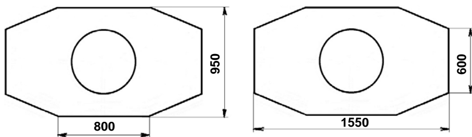
Рис. 7. Размеры перекрытия колодца «ККСр-3М-10(80)».
