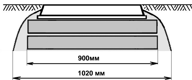
Рис. 14. Размеры (диаметры) опорных колец типа КО и бетонной обмазки. Вид на колодец «ККСр-3-80» сбоку.
