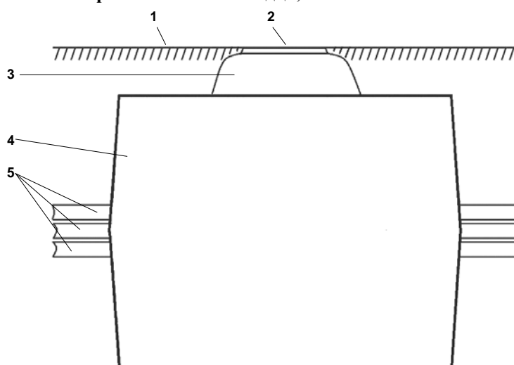
Рис. 2. Колодец «ККСр-3М-10(80)», как подземное сооружение: 1 – уровень земли или асфальта на тротуаре; 2 – чугунный люк; 3 – горловина в бетонной обмазке; 4 – корпус (верхний и нижний элементы); 5 – блок вводимых каналов.
