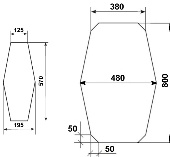
Рис. 2.2. Размеры технологического отверстия и участка с тонкой неармированной стенкой на торцевой стене колодца «ККСр-3М-10(80)».
