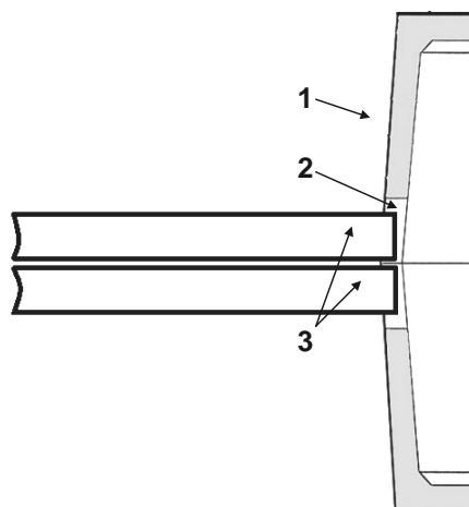
Рис. 11. Ввод труб в колодец «ККСр-3М-10(80)»: 1 – торцевая стена колодца; 2 – проём в торцевой стене; 3 – хризотилцементные (асбестоцементные) трубы.
