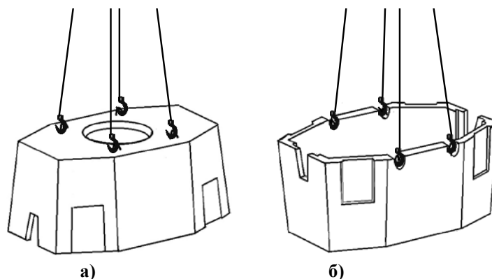
Рис. 10. Строповка элементов «ККСр-3М-10(80)»: а – верхнего элемента; б – нижнего элемента.
