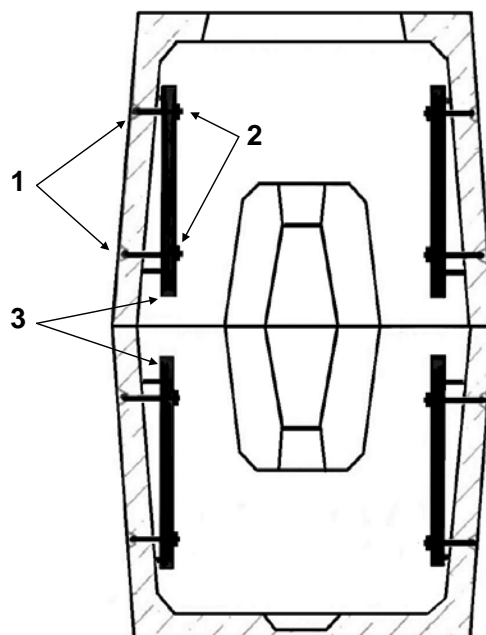
Рис. 3.1. Кронштейны «УККП-60» в колодце «ККСр-3М-10(80)»: 1 – ерши с резьбой в отверстиях боковой стены колодца; 2 – гайки и шайбы; 3 – кронштейны «УККП-60».
