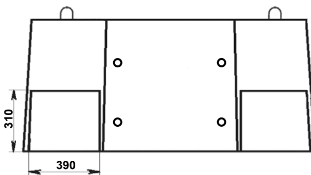
Рис. 8. Размеры ниш на примере верхнего элемента колодца «ККСр-3М-10(80)». На нижнем элементе ниши такого же размера.
