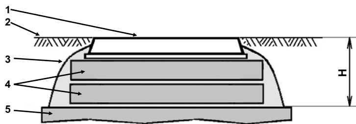
Рис. 13. Расстояние от перекрытия колодца до уровня земли (асфальта) – H: на тротуаре и газоне – не менее 250 мм; на проезжей части – не менее 330 мм: 1 – люк чугунный; 2 – уровень земли на газоне, асфальта на тротуаре или дорожного покрытия на проезжей части улиц; 3 – обмазка бетоном со щебнем; 4 – опорные кольца типа КО; 5 – перекрытие колодца «ККСр-3М-10(80)».
