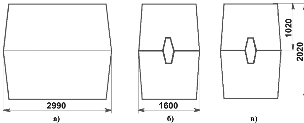
Рис. 5. Габаритные размеры колодца «ККСр-5-80»: а - вид сбоку; б и в – виды с торца.
