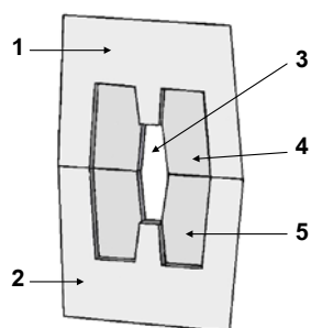
Рис. 2.1. Участок с тонкой неармированной стенкой на торцевой стене колодца «ККСр-5-80»: 1 – торцевая стена верхнего элемента; 2 – торцевая стена нижнего элемента; 3 – технологическое отверстие; 4 - участок с тонкой неармированной стенкой на верхнем элементе; 5 - участок с тонкой неармированной стенкой на нижнем элементе.
