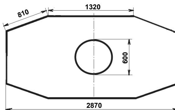
Рис. 6. Размеры перекрытия колодца «ККСр-5-80».
