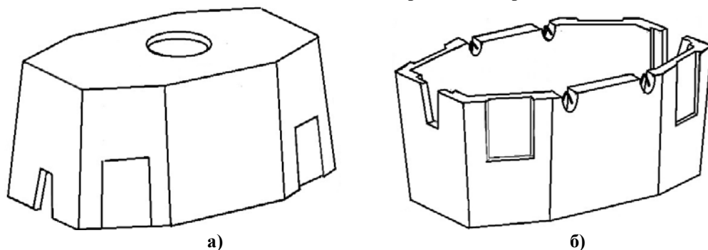
Рис. 1. Колодец «ККСр-5-80» как изделие по ТУ 45 1418-83: а – верхний элемент; б – нижний элемент.
