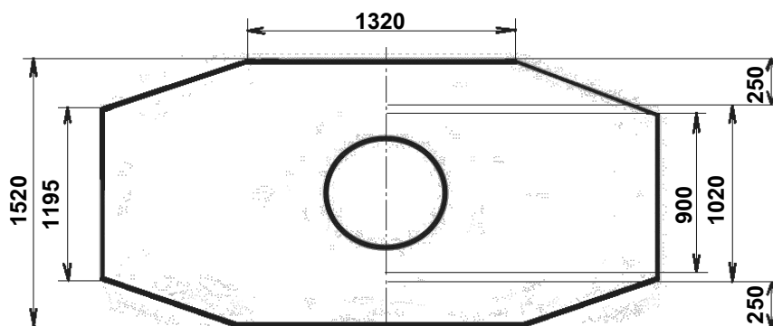
Рис. 7. Размеры перекрытия колодца «ККСр-5-80» с указанием диаметров опорных колец: 900 мм – кольца типа КО; 1020 мм – кольца КО-ЧП и КО-Ч.
