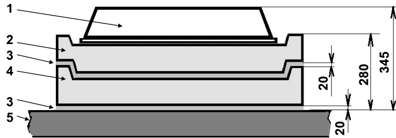
Рис. 13. Высота горловины с парой колец «КО-ЧП» и «КО-Ч»: 1 – люк чугунный типа «Т»; 2 – кольцо «КО-Ч»; 3 – слой бетона со щебнем; 4 – кольцо «КО-ЧП»; 5 – перекрытие колодца «ККСр-5-80».
