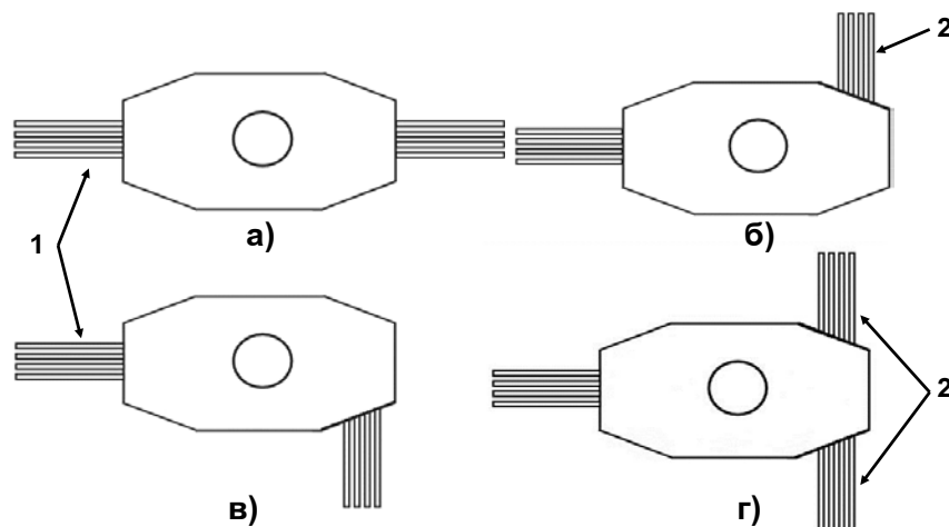
Рис. 3. Варианты использования колодца «ККСр-5-80»: 1 – вводимые каналы; 2 – ответвляющиеся каналы; а - проходной колодец; б, в – угловые колодцы; г - разветвительный колодец.
