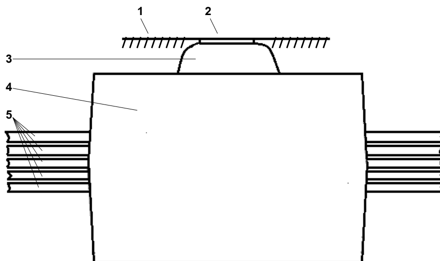
Рис. 2. Колодец «ККСр-5-80» как подземное сооружение: 1 – уровень земли или асфальта; 2 – чугунный люк; 3 – бетонная обмазка горловины; 4 – корпус колодца в сборе; 5 – вводимые каналы, 24 трубы.
