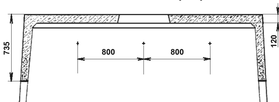
Рис. 8. Размеры ниш на примере верхнего элемента колодца «ККСр-5-80». На нижнем элементе ниши такого же размера.
