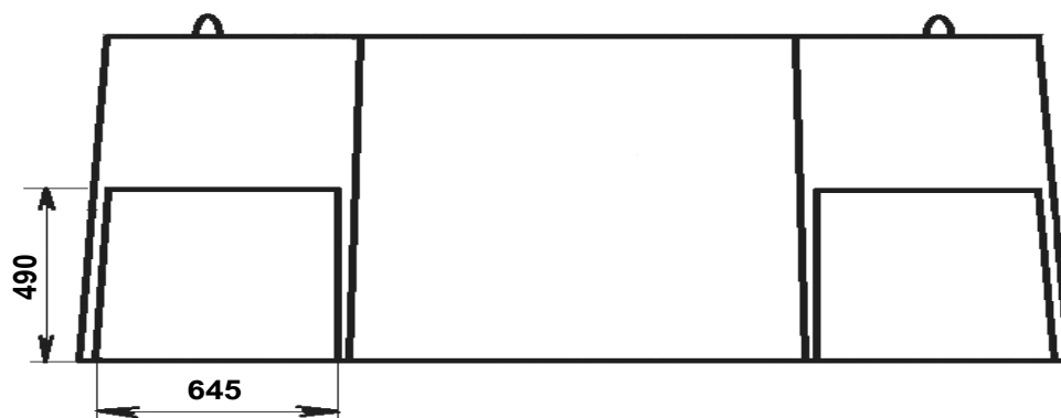
Рис. 8. Размеры ниш на примере верхнего элемента колодца «ККСр-5-80». На нижнем элементе ниши такого же размера.
