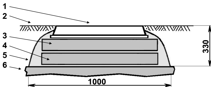
Рис. 12. Горловина с кольцами типа КО и люком типа «Т»:
