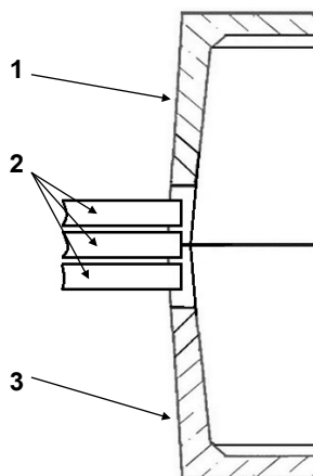
Рис. 10. Ввод труб в колодец «ККСр-5-80»:
