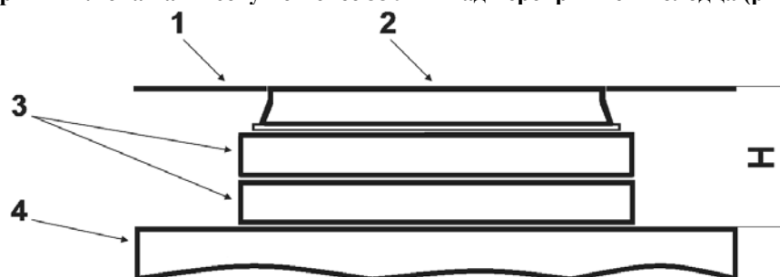
Рис. 12. Заглубление колодца «ККСр-2,5-10(80)» при установке на тротуаре или газоне, вид на колодец сбоку:
