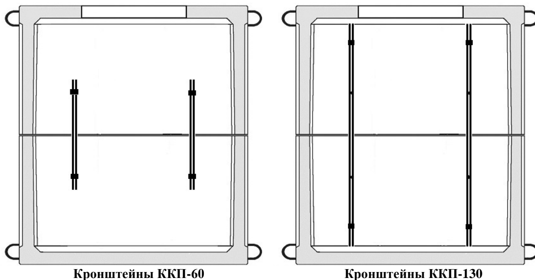
Рис. 1. Боковые стены колодца «ККСр-2-10(80) (вибро)» с установленными кронштейнами. В процессе эксплуатации колодца на кронштейны могут устанавливаться консоли типа «ККЧ».
