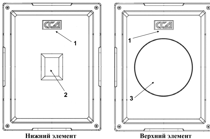
Рис. 2. Внутренние детали элементов колодца «ККСр-2,5-10(80)»: 1 – логотип компании ССД; 2 – приямок для стока воды; 3 – круглое отверстие для люка, диаметр – 600 мм.
