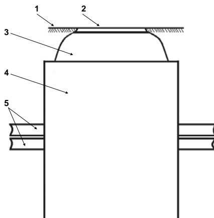
Рис. 6. Колодец «ККСр-2,5-10(80)» как подземное сооружение: 1 – уровень земли или дорожного покрытия; 2 – люк чугунный; 3 – горловина в бетонной обмазке; 4 – колодец в сборе; 5 – вводимые каналы.
