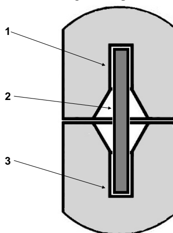
Рис. 11. Фиксатор смещения в соединённых элементах колодца:
