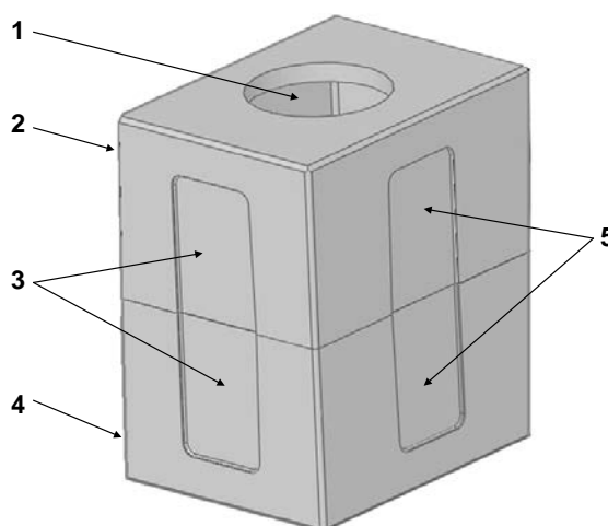
Рис. 3. Детали колодца «ККСр-2,5-10(80)» в сборе: 1 – круглое отверстие для люка, диаметр 600 мм; 2 – верхний элемент; 3 – ниши на торцевой стене; 4 – нижний элемент; 5 – ниши на боковой стене.
