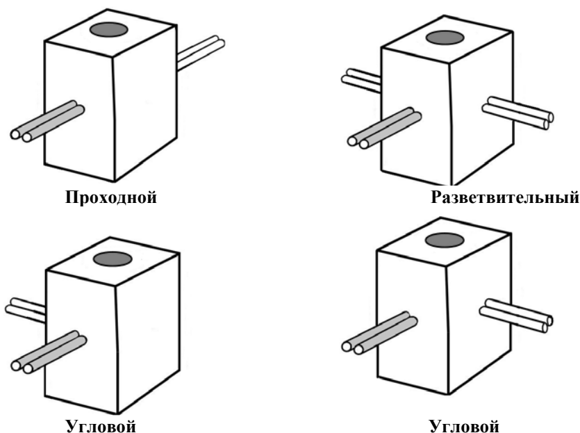
Рис. 7. Варианты использования колодца «ККСр-2,5-10(80)» в классических вариантах (для кабелей с медными жилами).
