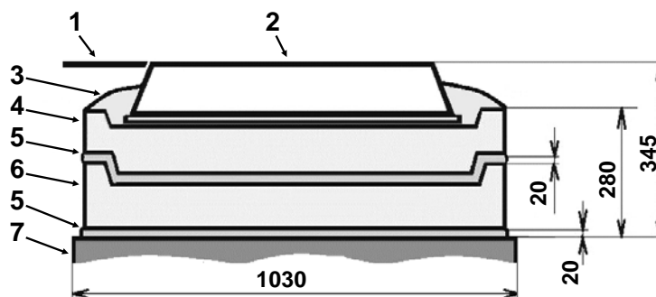
Рис. 14. Высота горловины с парой колец «КО-ЧП» и «КО-Ч», вид на колодец с торцевой стены:
